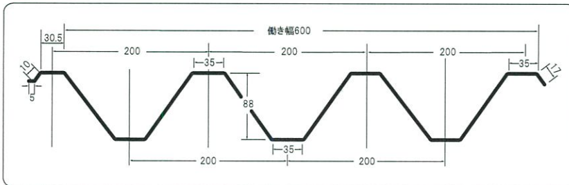
断面形状図
