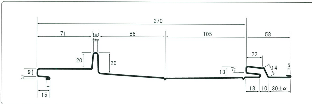
断面形状図
